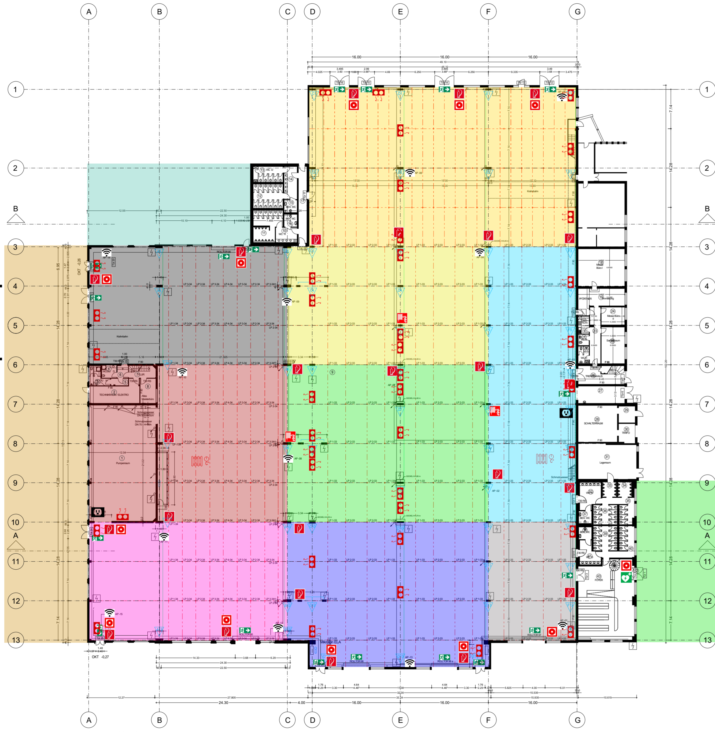
GRUNDRISS EG
